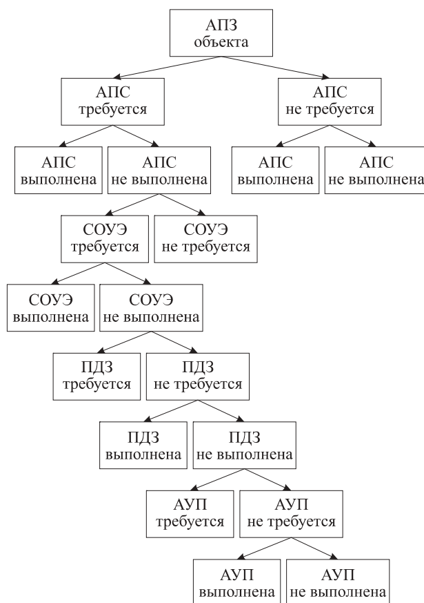
Дерево событий
